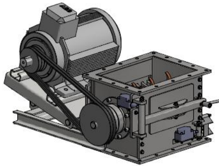
Lump Breaker (Lump Crusher)
